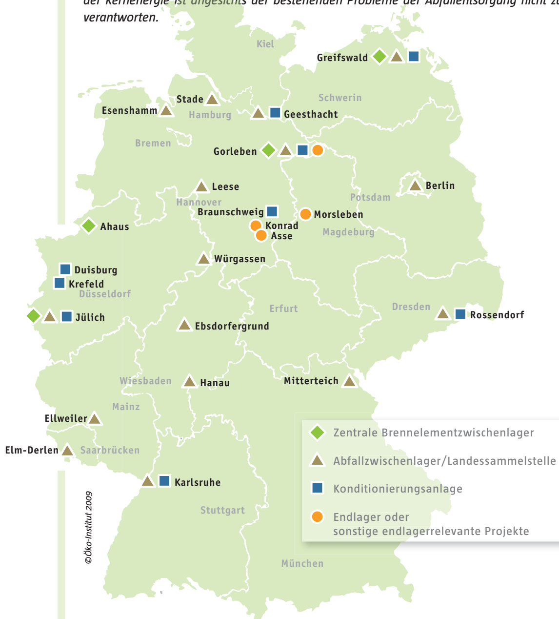
Bild 15: Entsorgungsanlagen in Deutschland (ohne dezentrale Brennelementzwischenlager an den Kernkraftwerks-Standorten)
